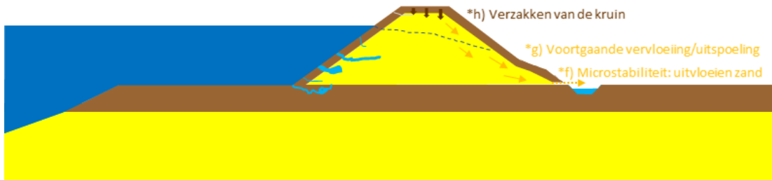
Figuur 2.14 Buitendijkse graverijen: vervolg van faalpad microstabiliteit
