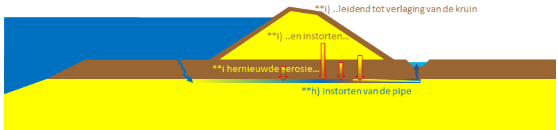
Figuur 2.19 Buitendijkse graverij, faalpad met falen door herhaald instorten van de pipe, tot aan kruinverlaging
