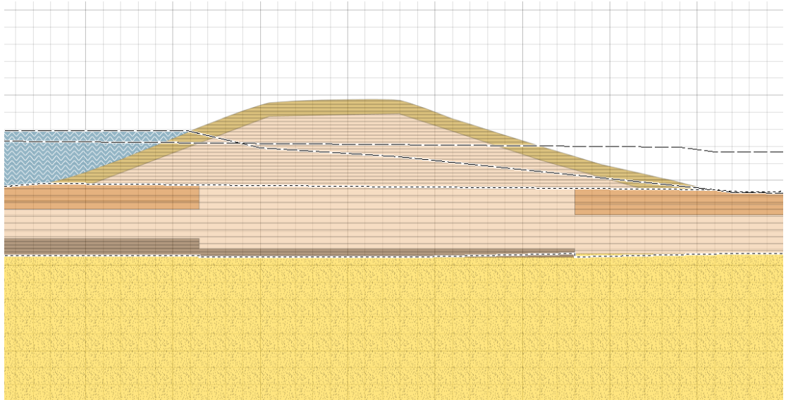
Figuur 2.5 Dwarsprofiel DR172.+09.0 (tijdens MHW) (de afstand tussen 2 gridlijnen bedraagt 1 m)
