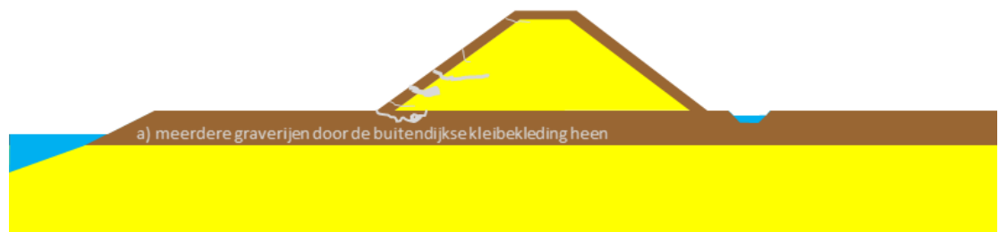
Figuur 2.11 Buitendijkse graverijen: eerste stap bij laag water
